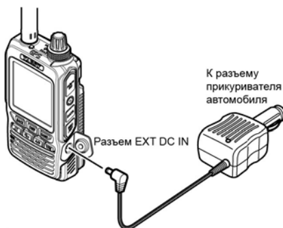
Адаптер внешнего источника питания с разъемом прикуривателя автомобиля. SDD-13 (опция)
